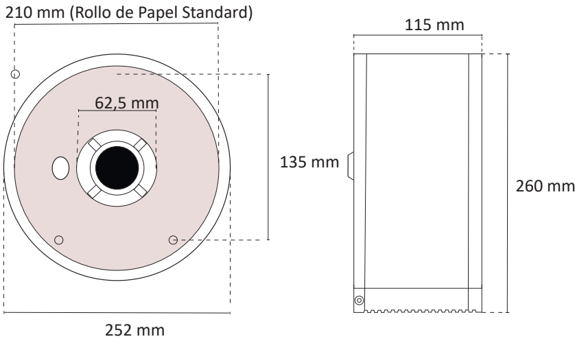
Esquema Válido para Códigos 031600300/400
