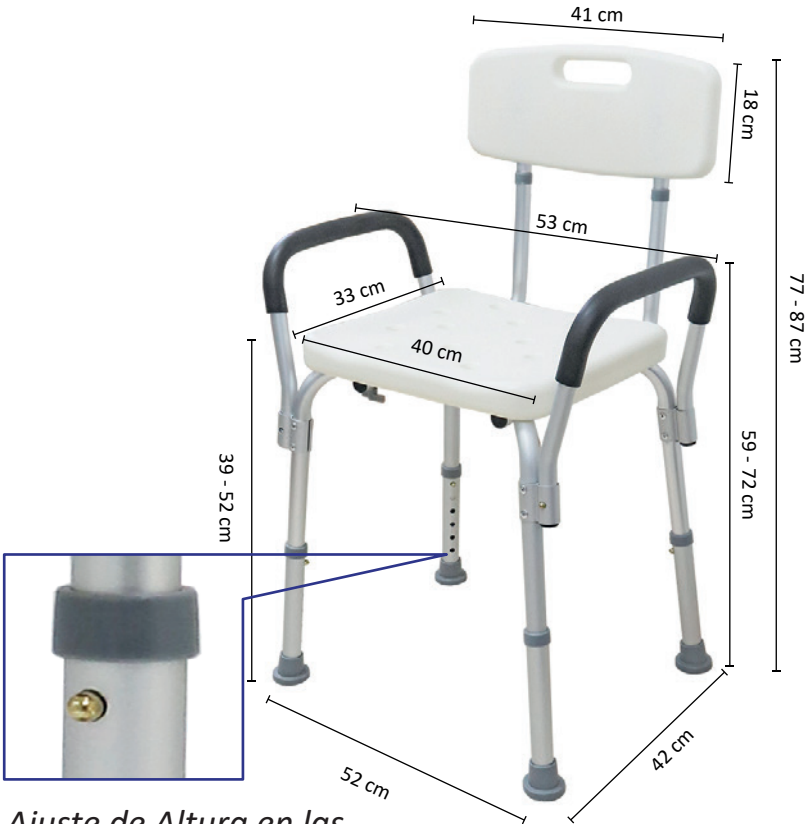
Ajuste de Altura en las Cuatro Patas (41 - 53 cm)
