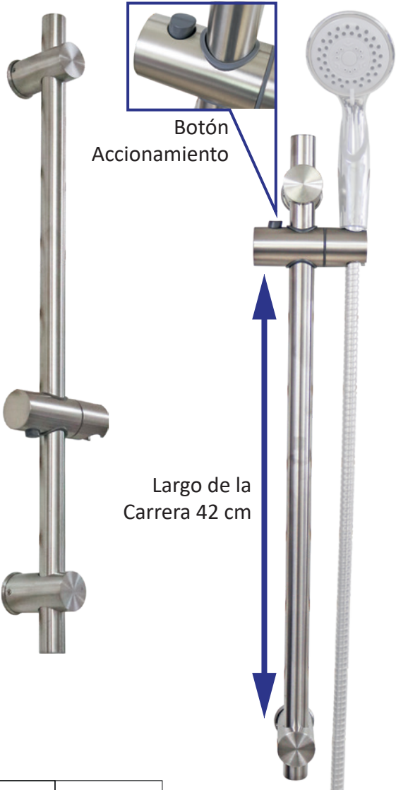
Barra Ducha Deslizable Inox 021000601
