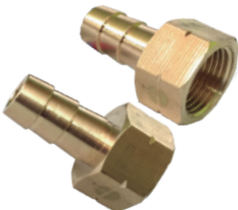
Cachimbo Recto HI 3/8" Izq. c/Espiga de 3/8" 113422081 113422083 (c/golilla y Abrazadera en Bolsa)
